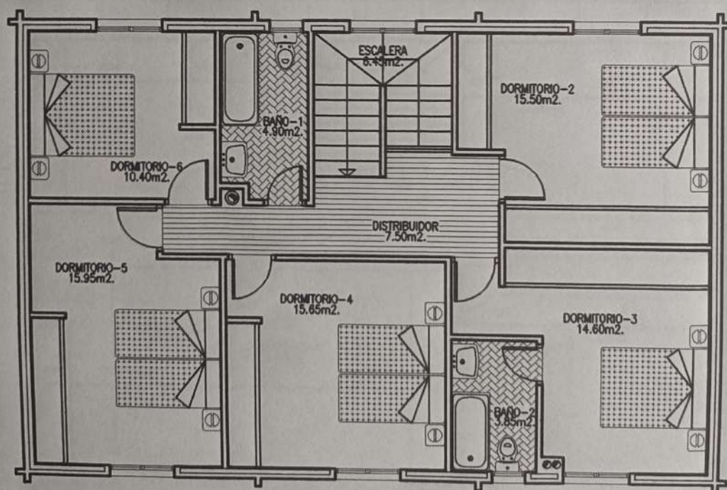
PLANTA PRIMERA
