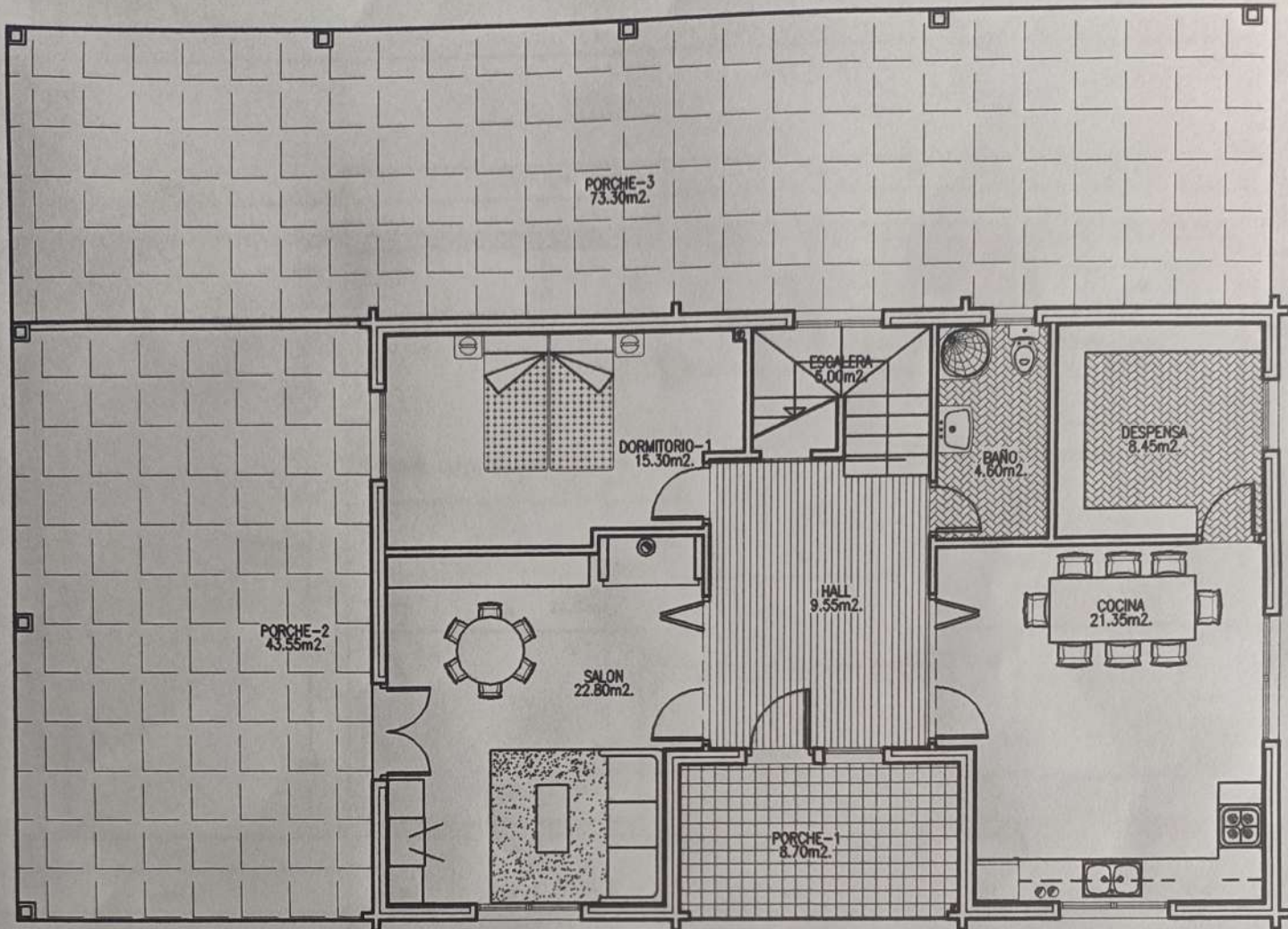
PLANTA BAJA
