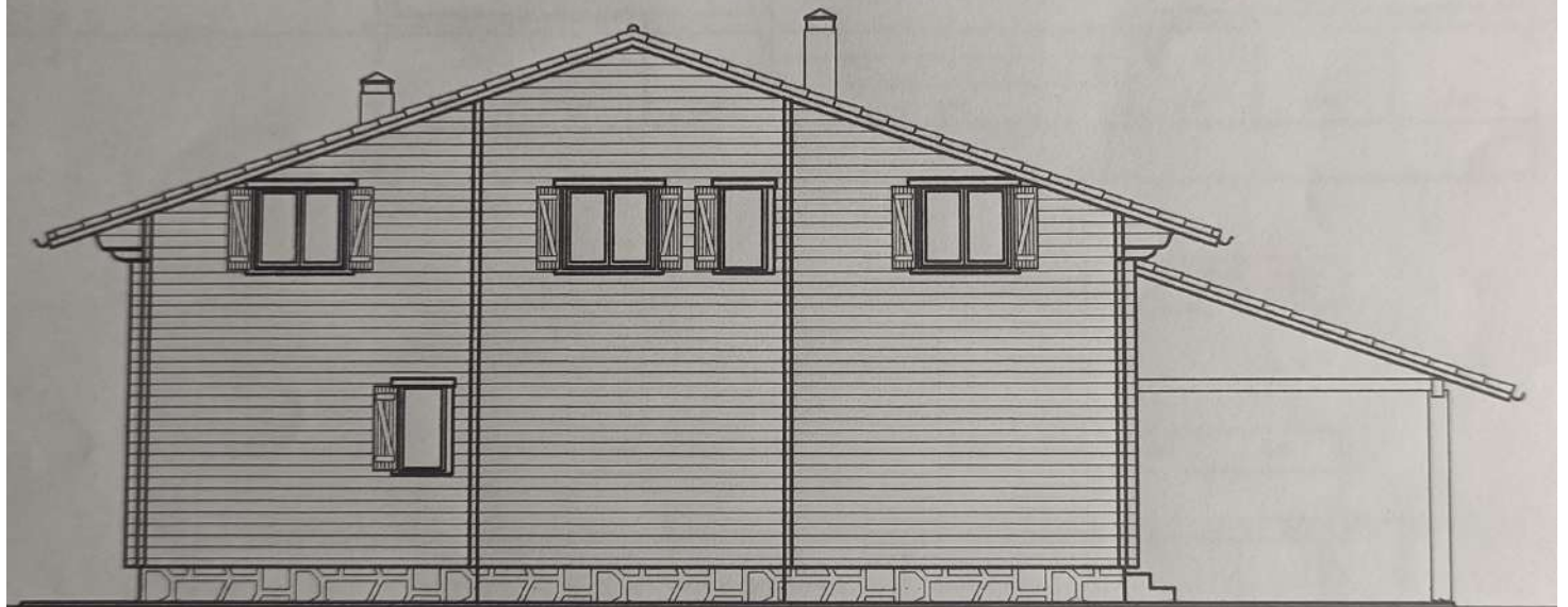
ALZADO POSTERIOR
